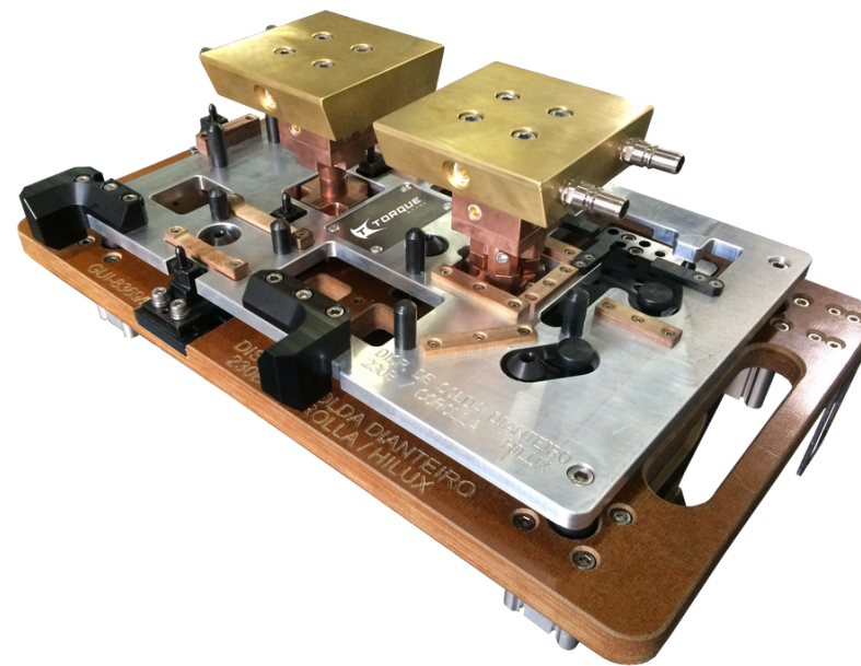
DISPOSITIVO DE SOLDA
