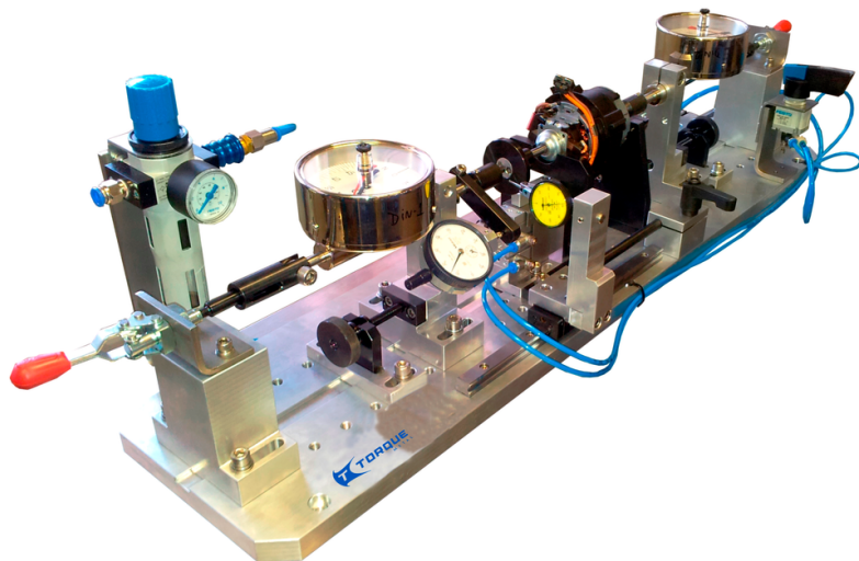
DINAMÔMETRO DE CALIBRAÇÃO
