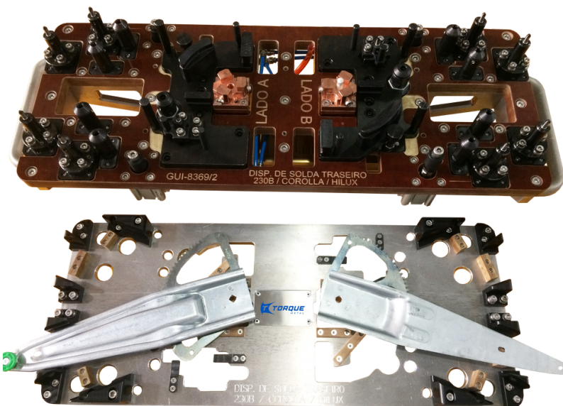
DISPOSITIVO DE SOLDA
