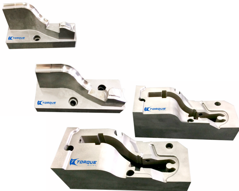
MATRIZ DE REBARBAÇÃO
