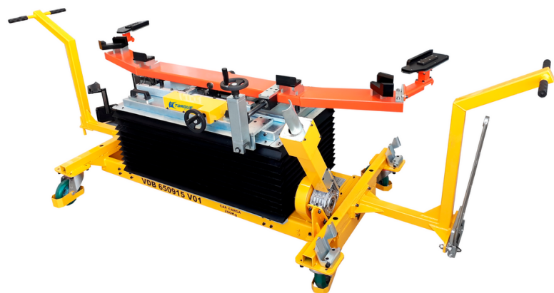
PRÉ-MONTAGEM PARA-CHOQUE
