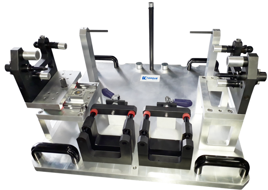
BERÇO DE MEDIÇÃO EM 3D
