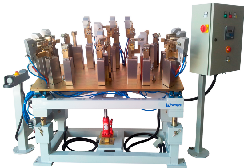
DISP. AUTOMATIZADO PARA ARAME DE BANCO
